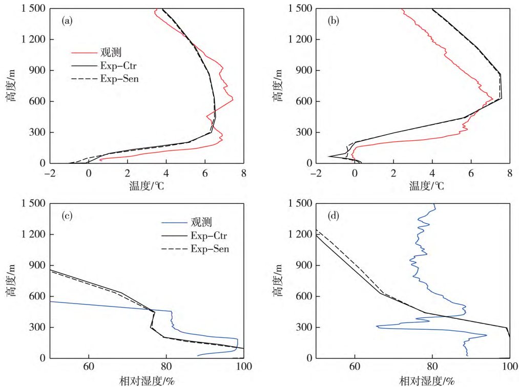
图 3 垂直结构对比 (a. 25 日 23 时温度 b. 26 日 23 时温度 c. 25 日 23 时相对湿度 d. 26 日 23 时相对湿度; 红色实线为探空观测温度, 单位: ^{\circ}\text{C} ; 蓝色实线为探空观测相对湿度, 单位: %; 黑色实线为 Exp-Ctr 试验结果, 黑色虚线为 Exp-Sen 试验结果)
