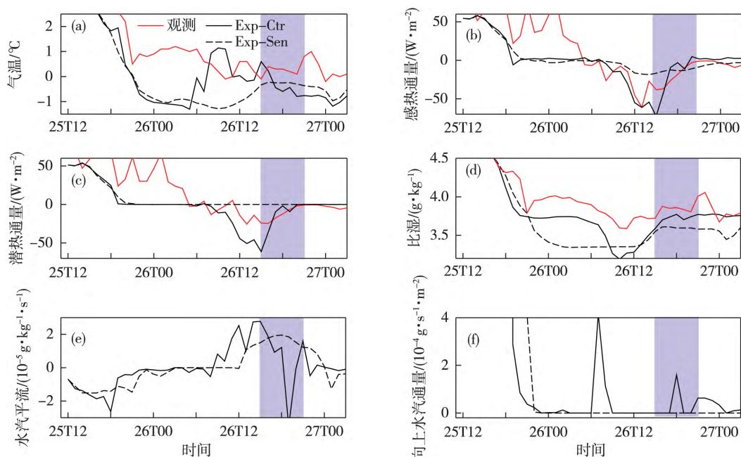
图 5 气温 (a, 单位: ^{\circ}\text{C} )、感热通量 (b, 单位: \text{W} \cdot \text{m}^{-2} )、潜热通量 (c, 单位: \text{W} \cdot \text{m}^{-2} )、比湿 (d, 单位: \text{g} \cdot \text{kg}^{-1} )、水汽平流 (e, 单位: 10^{-5} \text{g} \cdot \text{kg}^{-1} \cdot \text{s}^{-1} )、向上水汽通量 (f, 单位: 10^{-4} \text{g} \cdot \text{s}^{-1} \cdot \text{m}^{-2} ) 时间变化序列对比 (黑色实线为 Exp-Ctr 试验, 虚线为 Exp-Sen 试验, 红色实线为观测或通过观测计算的结果, 其中 b、c 的观测通量值被扩大为 4 倍; 紫色柱表示观测到的海雾时间)
