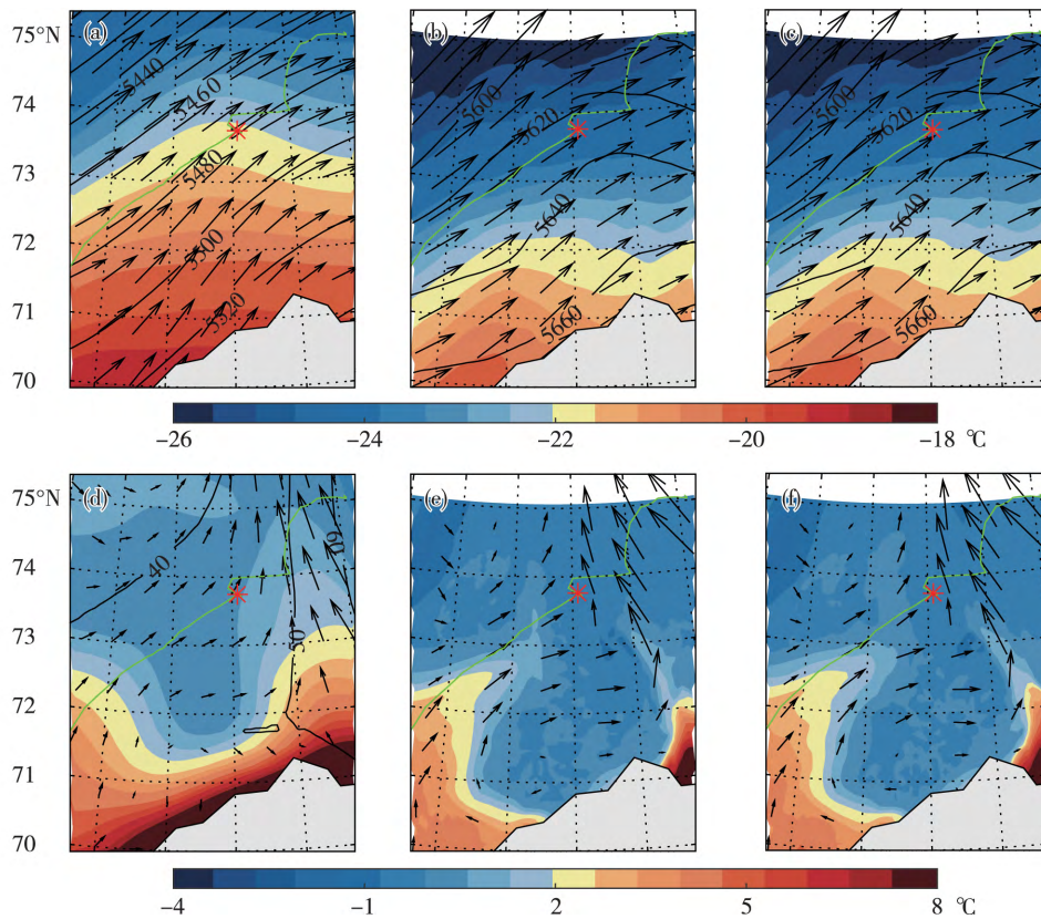
图 4 27 日 00 时空间各层环流场对比 ( a. ERA 500 hPa , b. Exp-Ctr 500 hPa , c. Exp-Sen 500 hPa , d. ERA 1 000 hPa , e. Exp-Ctr 1 000 hPa , f. Exp-Sen 1 000 hPa; 填色为温度 , 单位: ^{\circ}\text{C} ; 等值线为位势高度 , 单位: \text{gpm} ; 箭头为风矢量 , 绿线为航线 , 红星为此时船位置)
